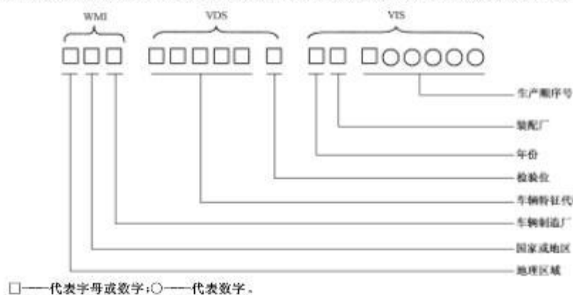
图1 年产量大于或等于1 000辆的完整车辆和/或非完整车辆制造厂车辆识别代号结构示意图
